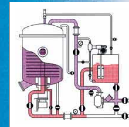
1. FORMAZIONE DEL PANNELLO DA FILTRARE / Unfiltered cake
