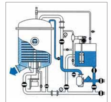
3. LAVAGGIO/ Washing / Acqua/ Water
